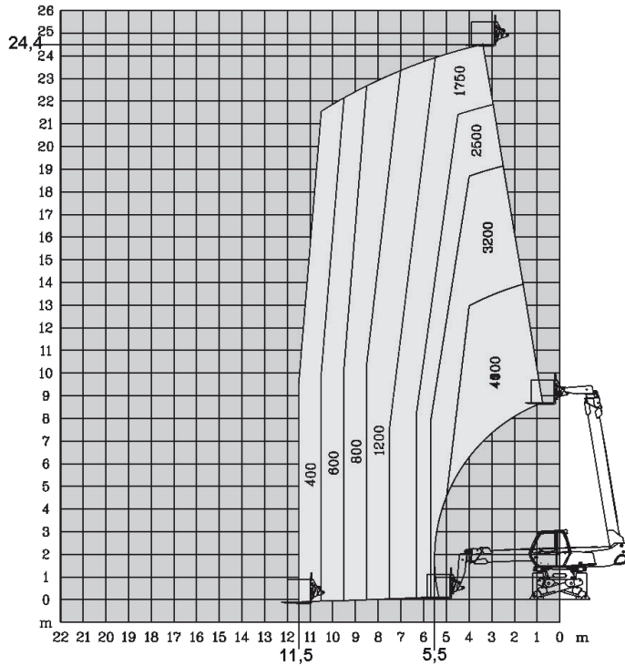
Lastfall 360°, 1/2 Abstützung, mit Gabeln
