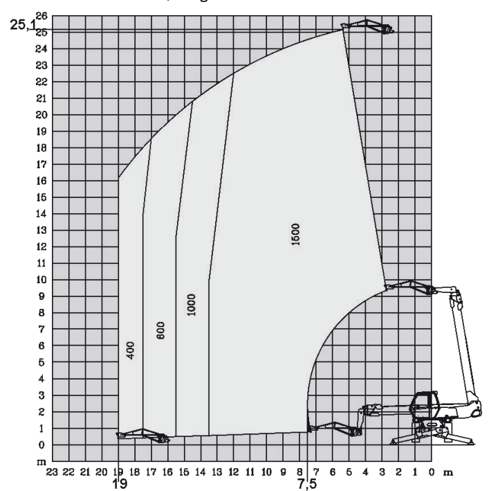
Lastfall 360°, abgestützt mit Jib P 1500
