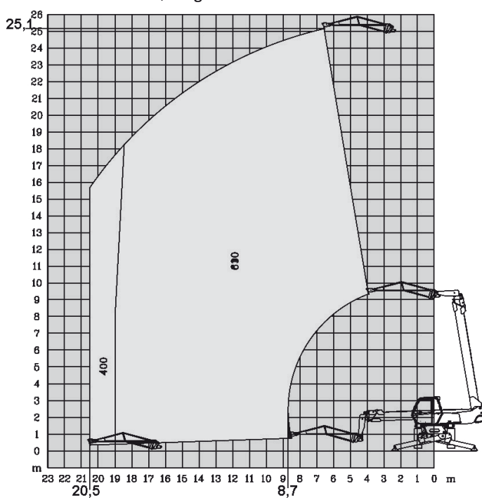
Lastfall 360°, abgestützt mit Jib P 600
