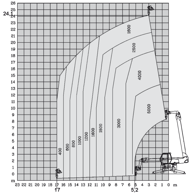
Lastfall 360°, abgestützt, mit Seilwinde 5T
