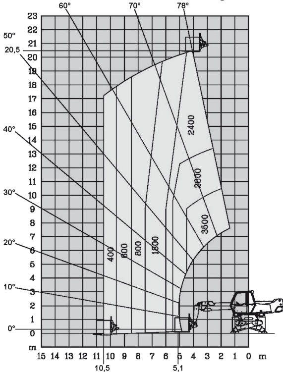
Lastfall 360°, 1/2 Abstützung, mit Gabeln
