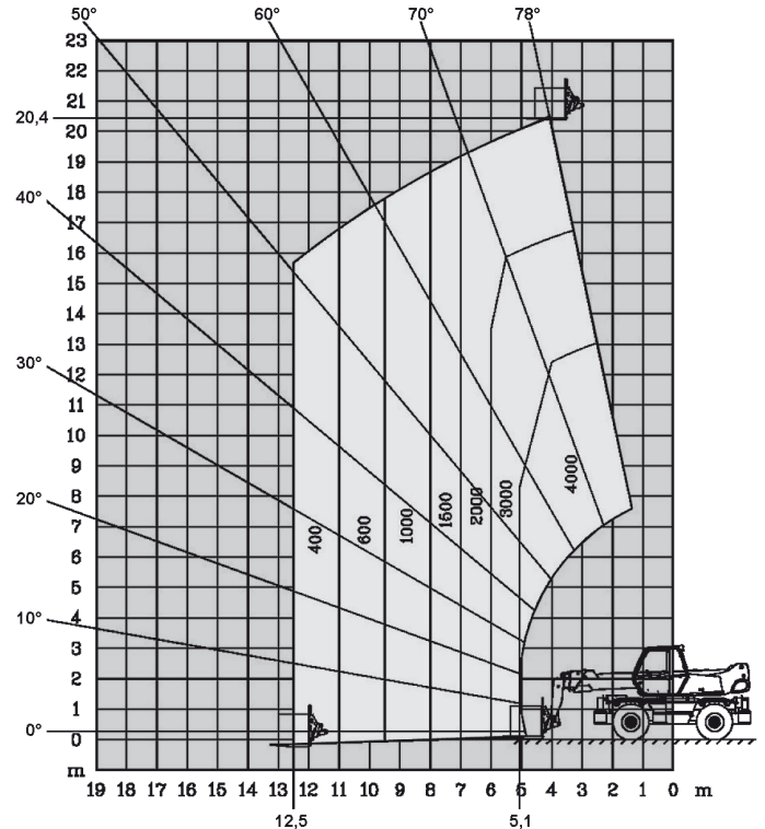
Lastfall frontal, auf Reifen, mit Gabeln
