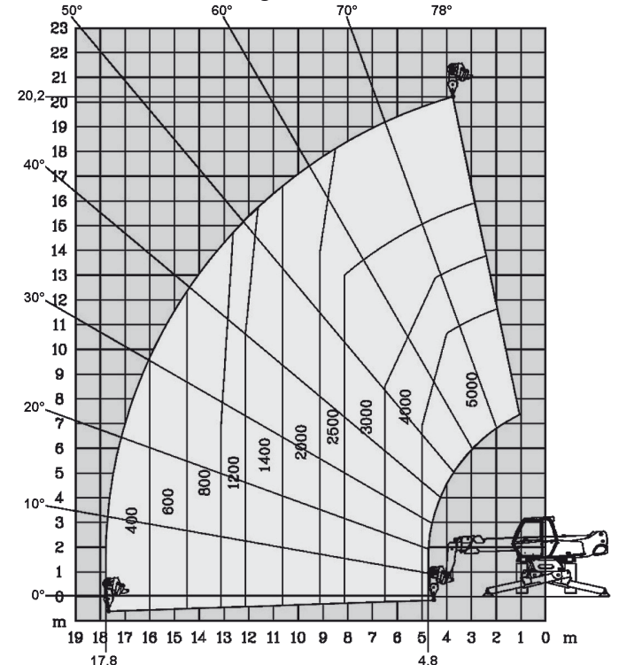
Lastfall 360°, abgestützt, mit Seilwinde 5T
