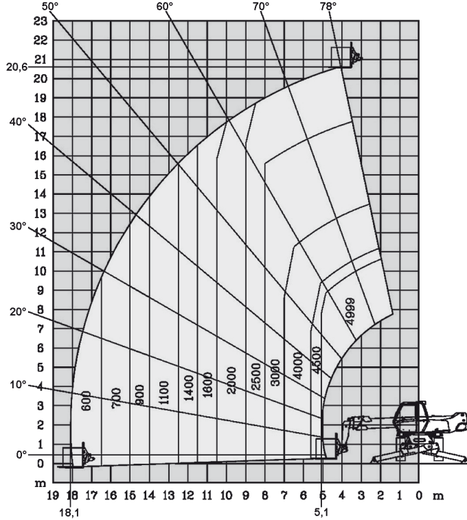
Lastfall 360°, abgestützt, mit Gabeln
