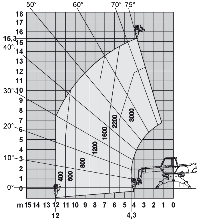
Lastfall 360°, abgestützt, mit Seilwinde 3T
