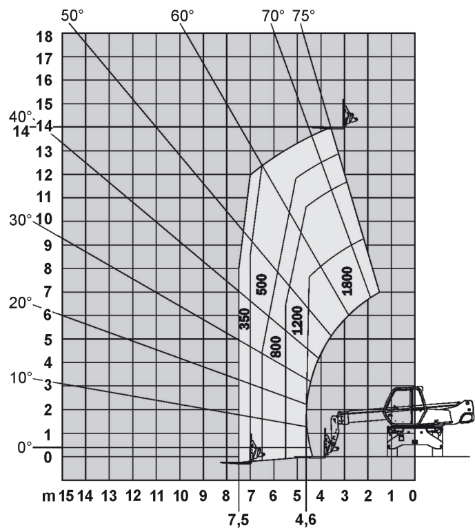
Lastfall 360°, auf Reifen, mit Gabeln
